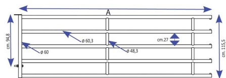
Barriera a 5 tubi con testata femmina
