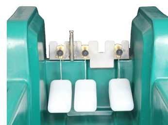
- 3 galleggianti ( 120 lt/min )
